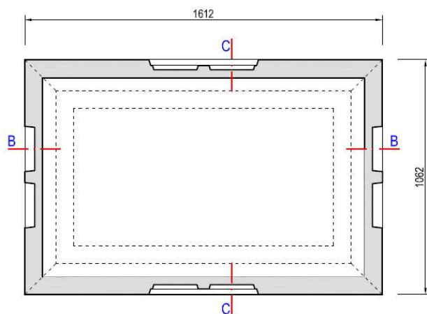
CORTE A-A
