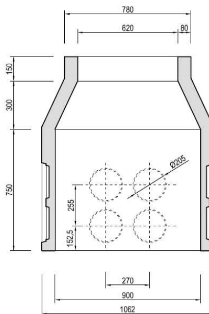
CORTE C-C
